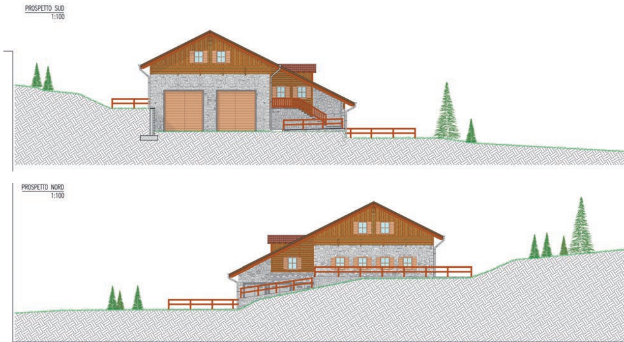
Prospetti del progetto di realizzazione dell'edificio Centrale
