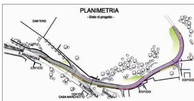
Planimetria dell'opera
